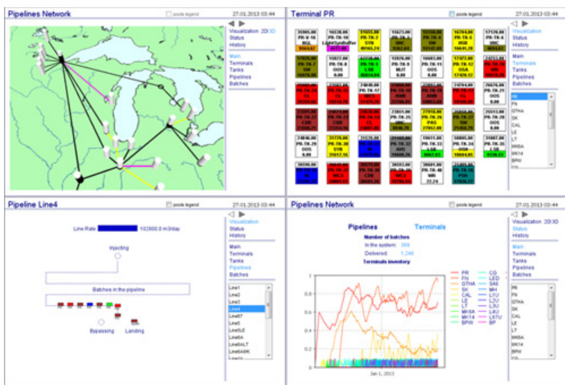
Интерфейс и анимация модели сети нефтепроводов
